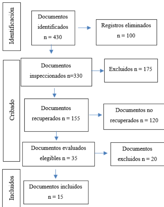
Figura 1. Método PRISMA
